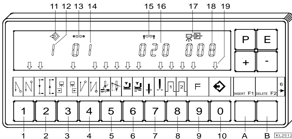
L'illustration suivante montre toutes les fonctions prévues pour la programmation de la couture TEACH IN.
